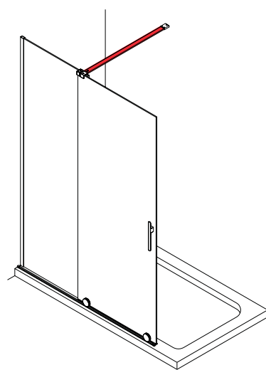
Mampara frontal (pag 454) compuesto por tensor frontal
